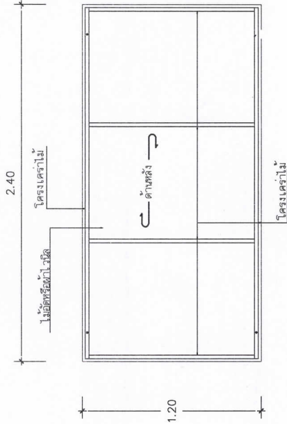
ด้านหลัง 1 : 25
